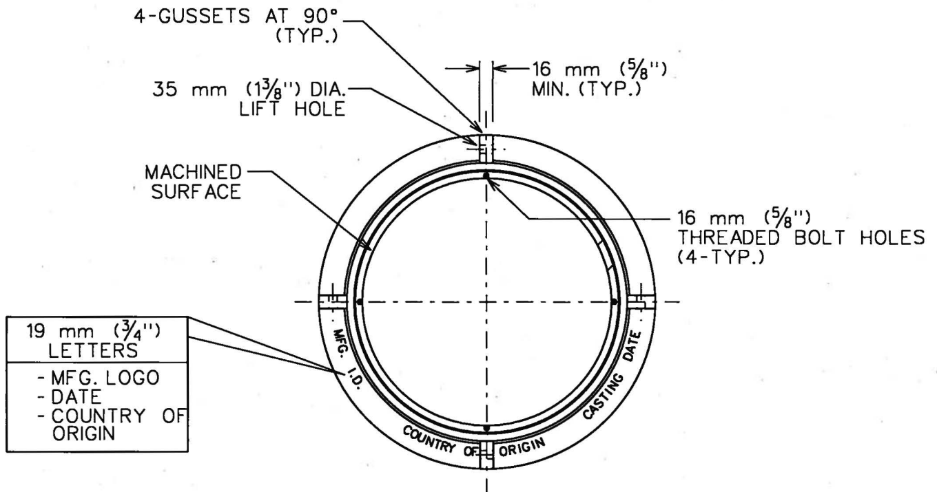
MANHOLE RING
