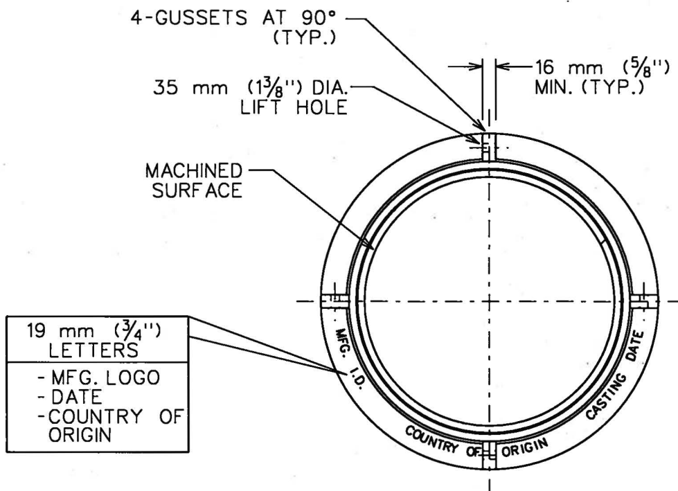
MANHOLE RING
