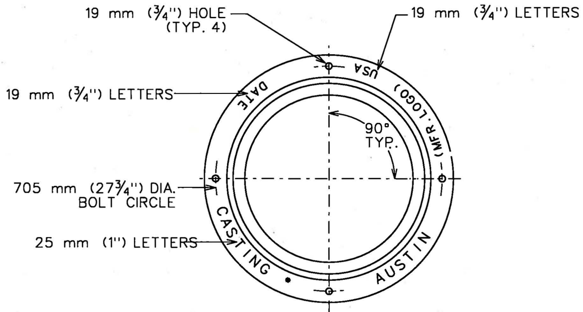
MANHOLE RING
