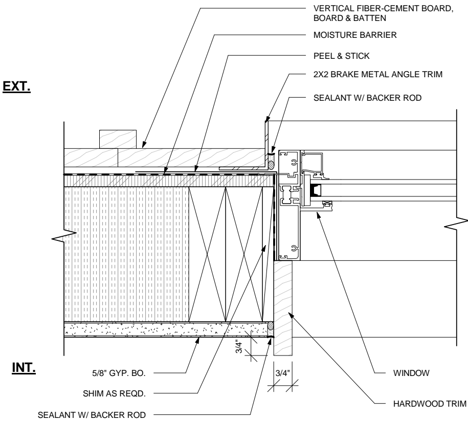
WINDOW TYP. JAMB
