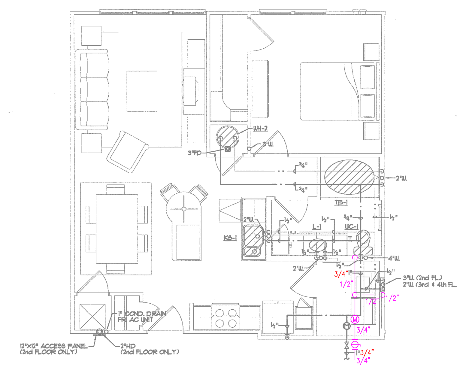
4 UNIT PLAN - A1A5 - PLUMBING SCALE: 1/4" = 1'-0"
