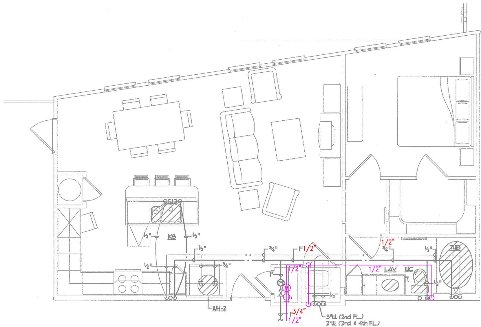
3 UNIT PLAN - A2 - PLUMBING SCALE: 1/4" = 1'-0"
