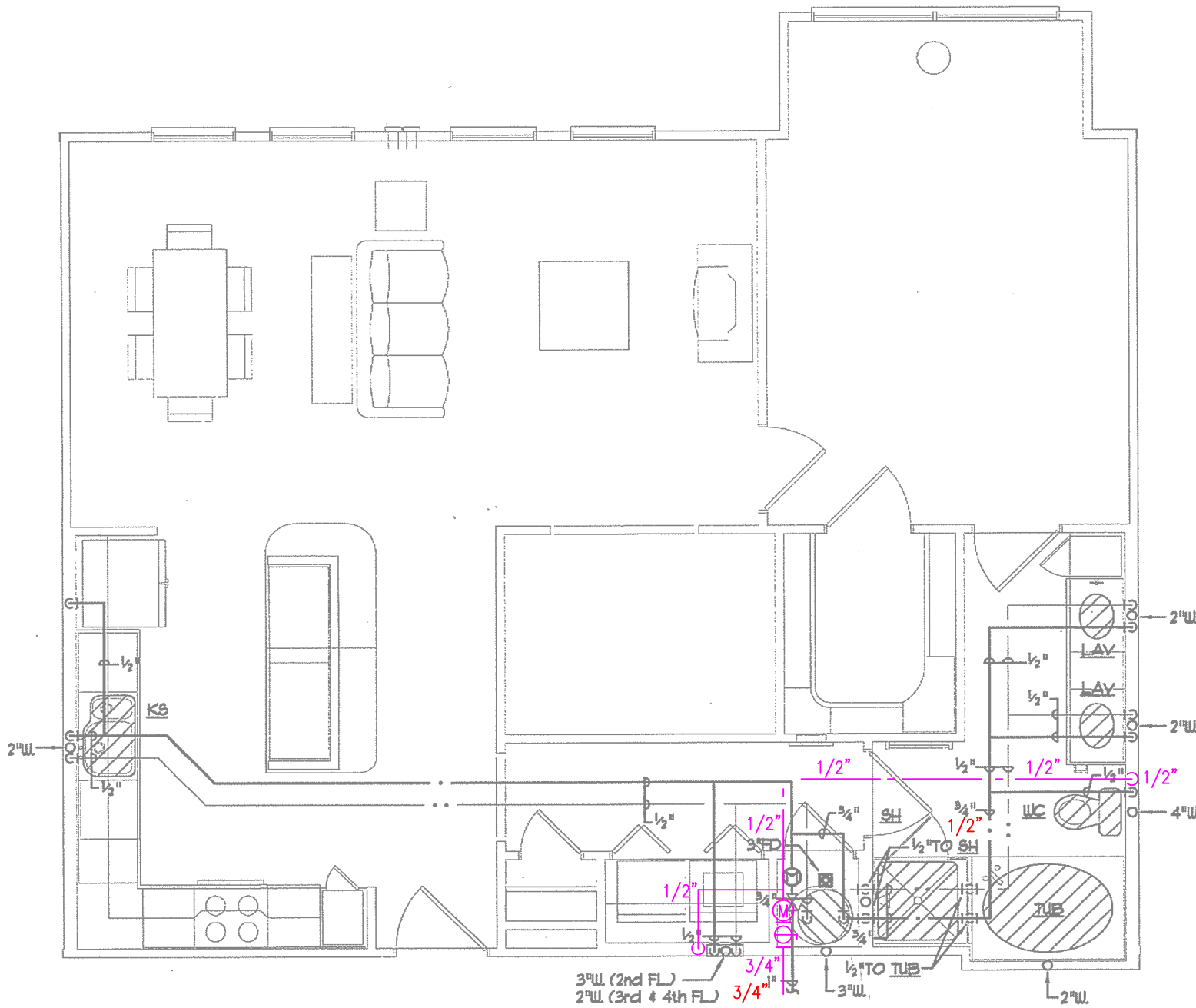
1 UNIT PLAN - A3 - PLUMBING SCALE: 1/4" = 1'-0"
