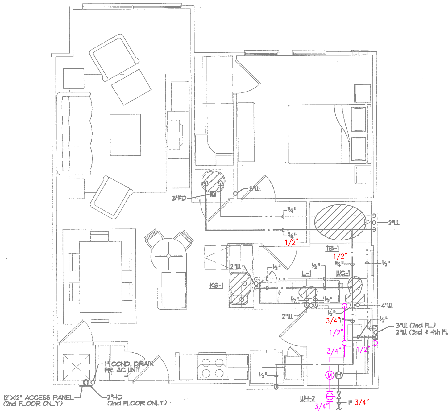
1 UNIT PLAN - A1 - PLUMBING SCALE: 1/4" = 1'-0"
