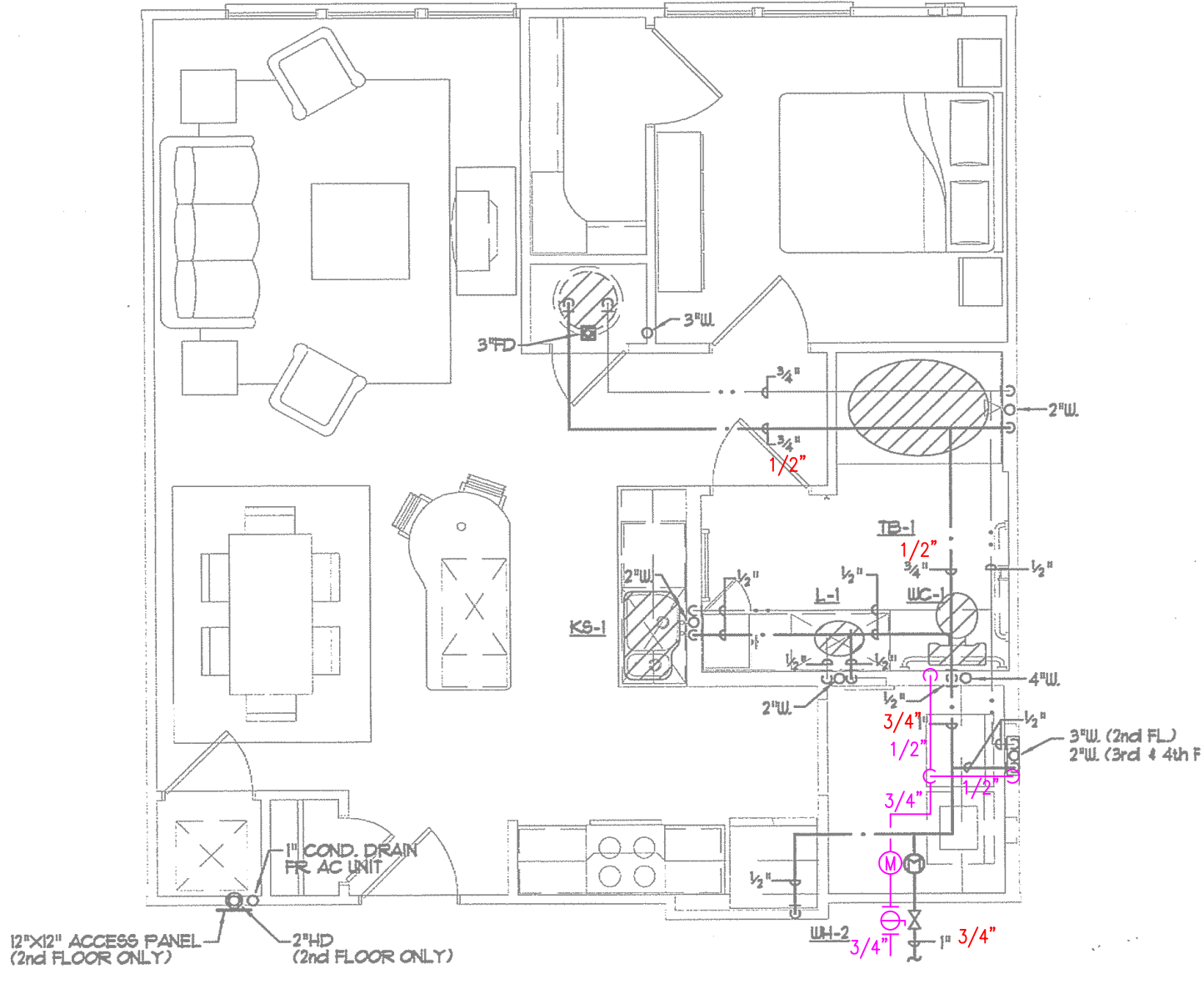
2 UNIT PLAN - A1 ANSI TYPE A - PLUMBING SCALE: 1/4" = 1'-0"
